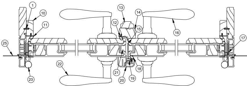
Jamb Detail
