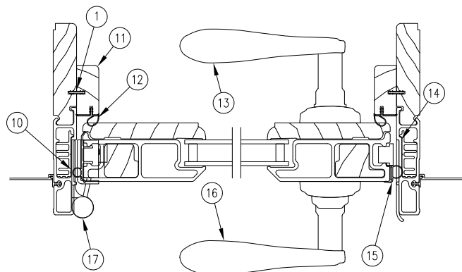
Jamb Detail
