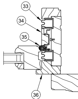
Jamb Detail
