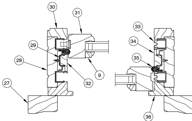
Jamb Detail
