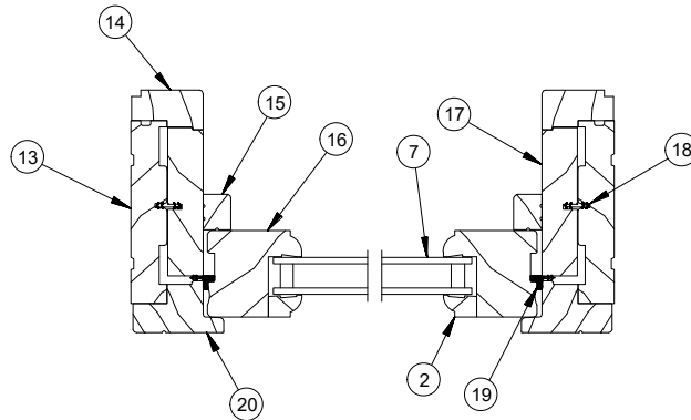
Jamb Detail
