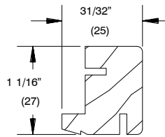
W6531 – Jamb Stop
