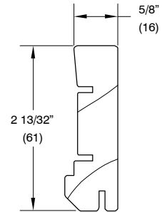
W11409 – Jamb Stop
