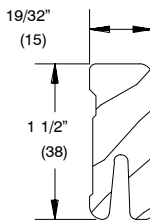
W2528 – Sill Liner (oak)
