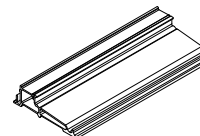
F256 – Ultrex Sill,* 4 9/16" Jamb
