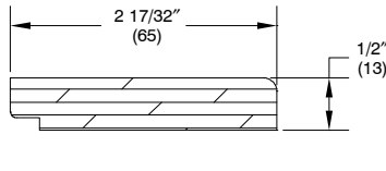
W7676 HJ Filler, IZ4
