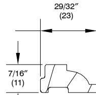
W9483 Glazing Stop, IZ3
