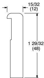
W7507 Sill Liner (Oak)
