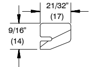
W7536 Jamb Liner
