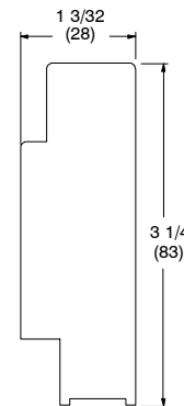
W7292 Center Jamb (OXO)
