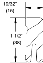
W2528 Sill Liner (Oak)
