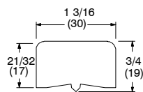
W1098 Interior Mull Casing (OOX or XO)
