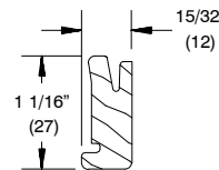
W8040 Panel Guide
