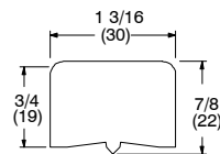
W1097 Exterior Mull Casing (OOX or XO)
