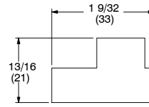
W7286 Stationary Panel Filler (OOX or XO)
