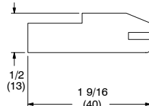
W7276 Jamb Liner
