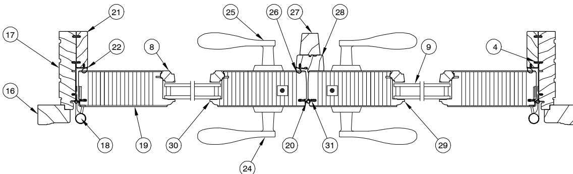
Jamb XX-R
