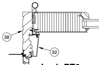
Jamb RT6
