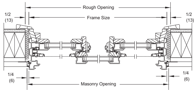
Triple Sash XOJ Operator Jamb
