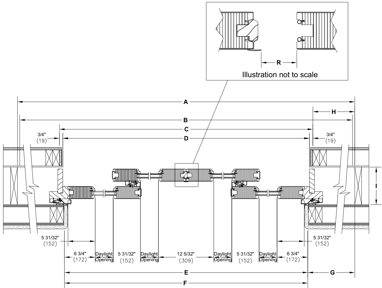
UWLSD PKT Tall Bottom Rail PXX - XXP
