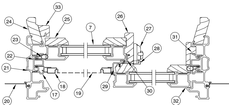
JAMB DETAIL
