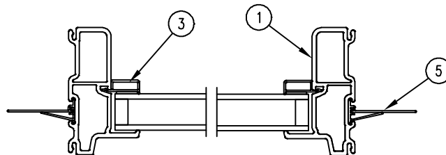
JAMB DETAIL
