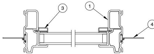
JAMB DETAIL
